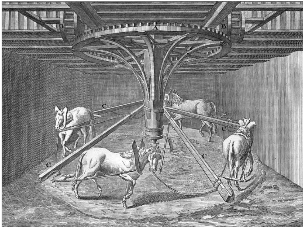
Fig. 2.- Molino de sangre, es decir, impulsado por fuerza animal ( Encyclopédie méthodique de Panckoucke, 1784).
